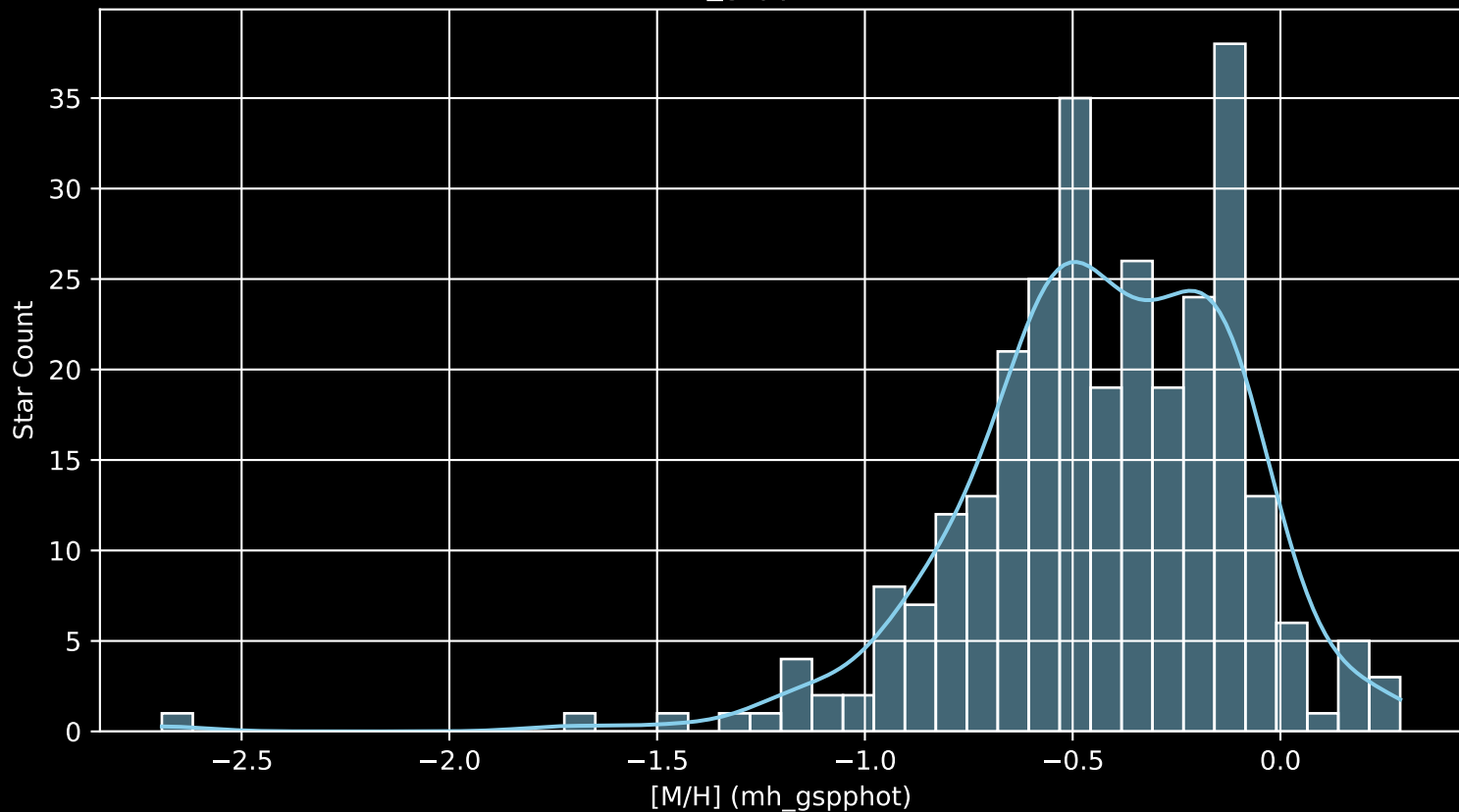
GALAH DR4 Field: [1012] [M/H] (mh_gspphot) (n= 288)
