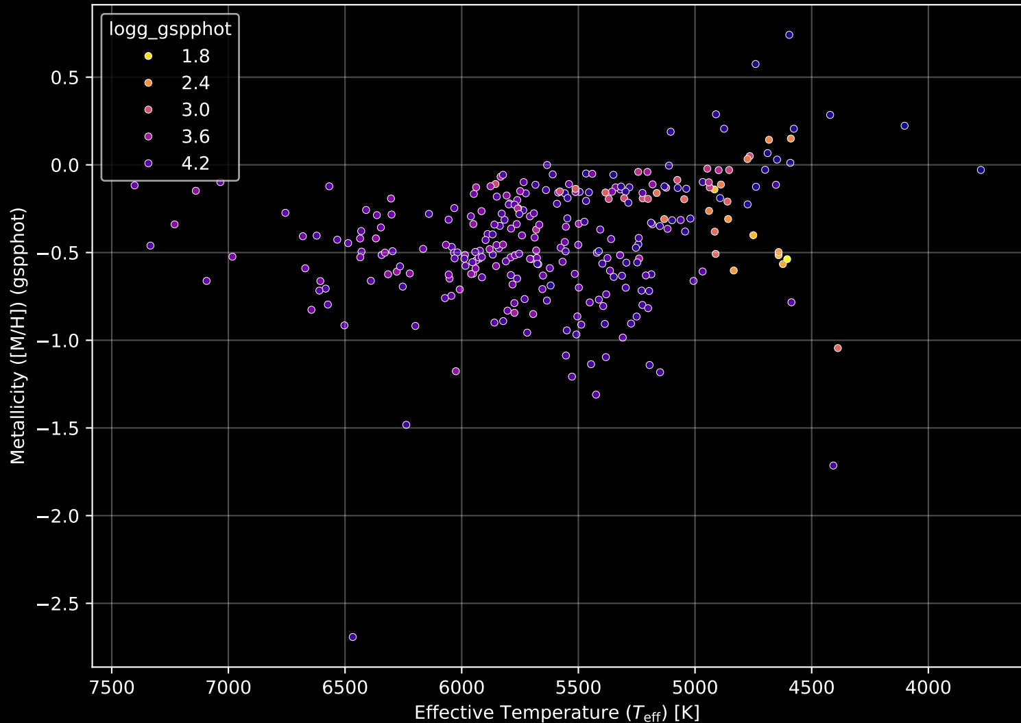
GALAH DR4 Field: [1012] Stellar Population Parameters (n= 290)
