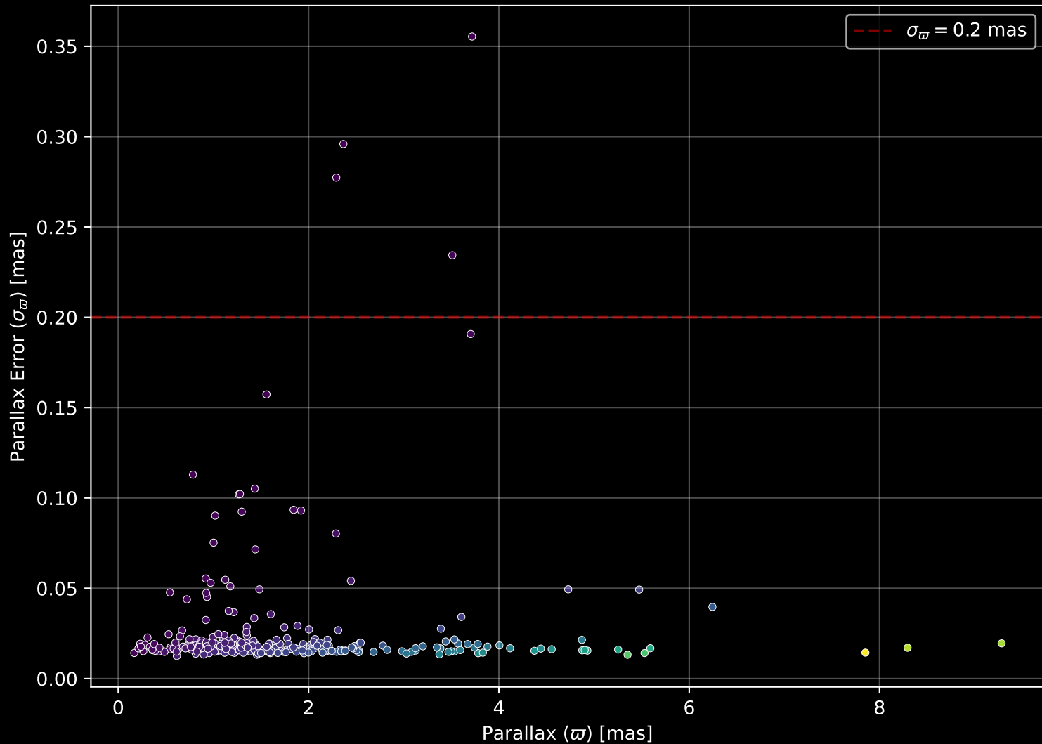
GALAH DR4 Field: [1012] Parallax Quality (n= 290)
