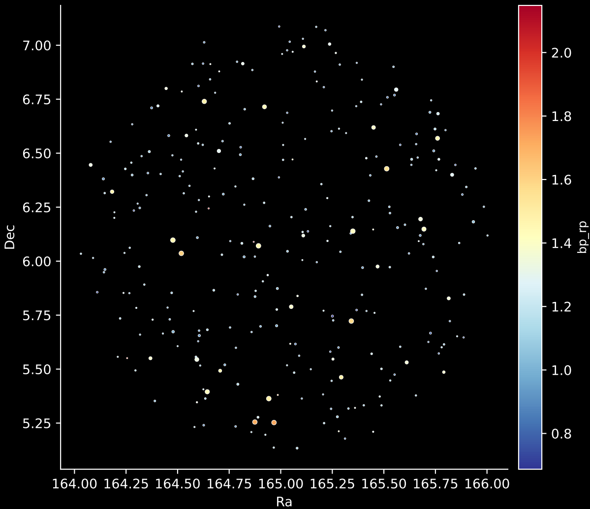
GALAH DR4 Field: [1012] Stars: 290
